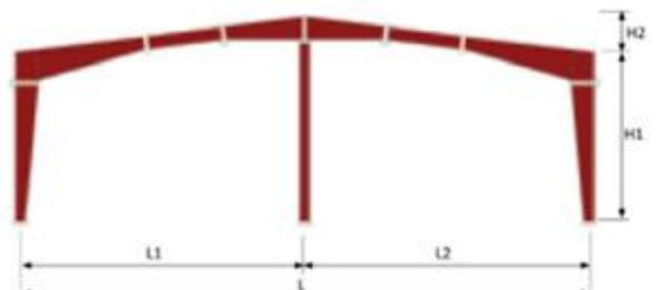
Khung thép định hình 2 nhịp
