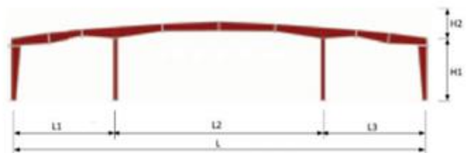
Khung thép định hình 3 nhịp
